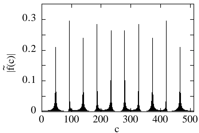
m=9 (QFT)
